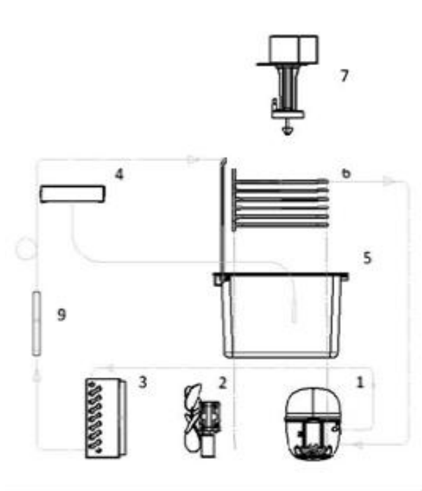
Рис. 1. Схема охладителя.
